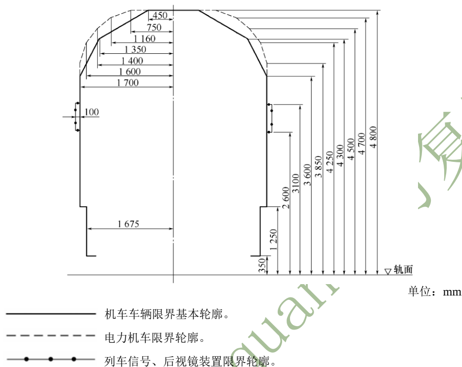
(1) 机车车辆上部限界图
