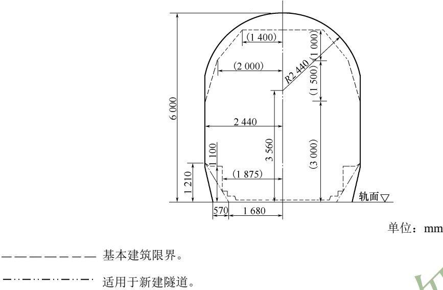
(4) 隧道建筑限界图（电力牵引区段）
