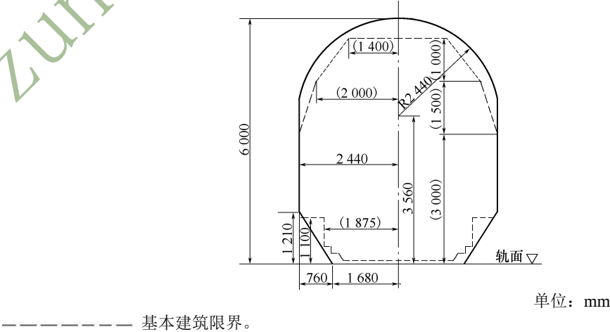
(5) 桥梁建筑限界图（内燃牵引区段）
