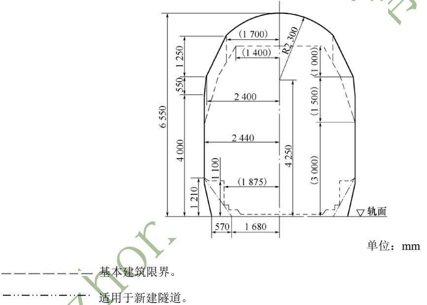
(5) 桥梁建筑限界图（内燃牵引区段）
