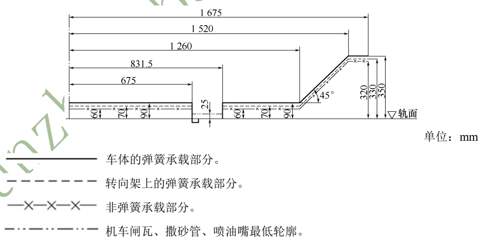
(2) 机车车辆下部限界图
